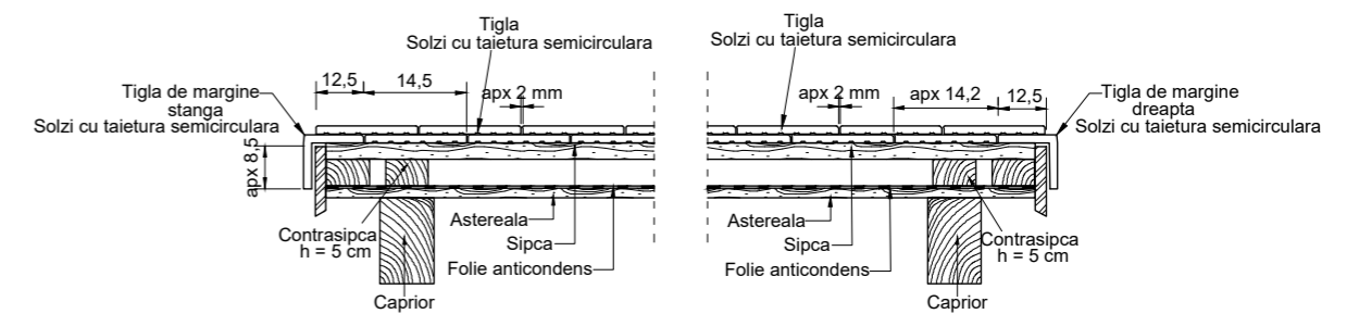
DETALIU ÎNCHIDERE MARGINE STÂNGA / DREAPTA
