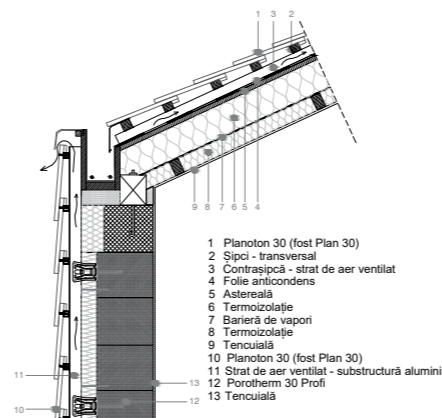
Detaliu 1
