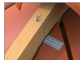
22 Clemă fixare țigă tăiată
