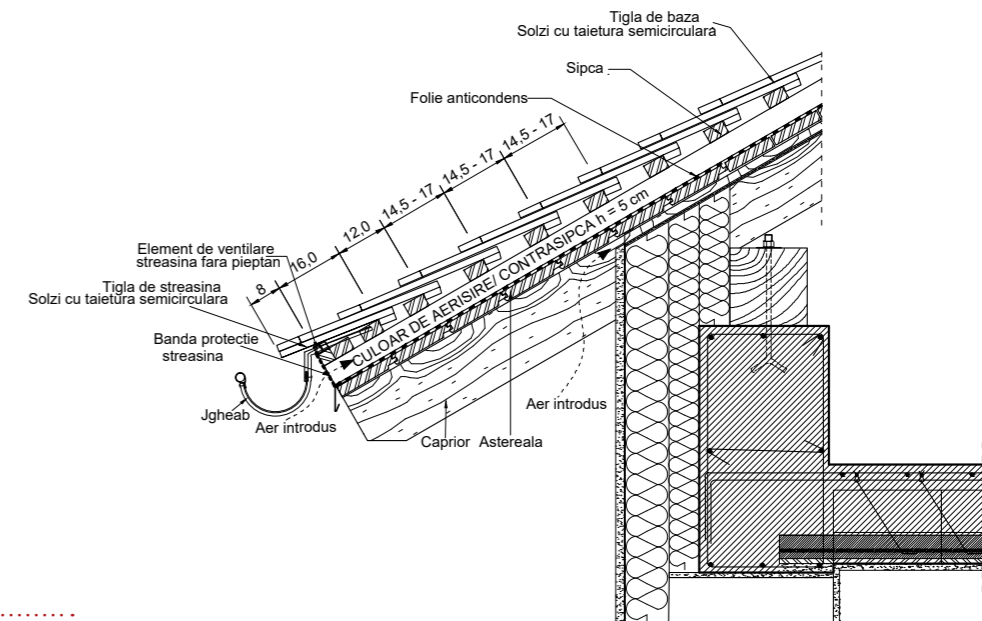
DETALIU STREAȘINĂ
