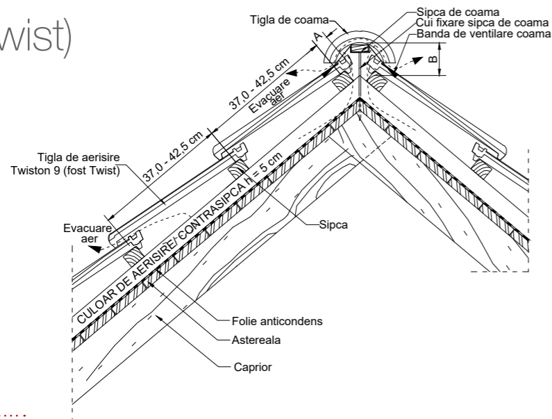
DETALIU COAMĂ
