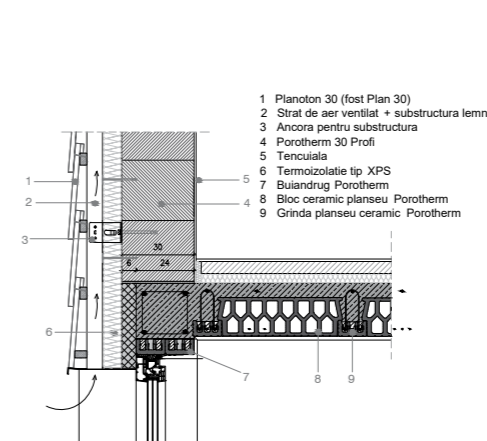
Detaliu 2
