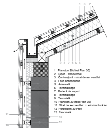
Detaliu 1
