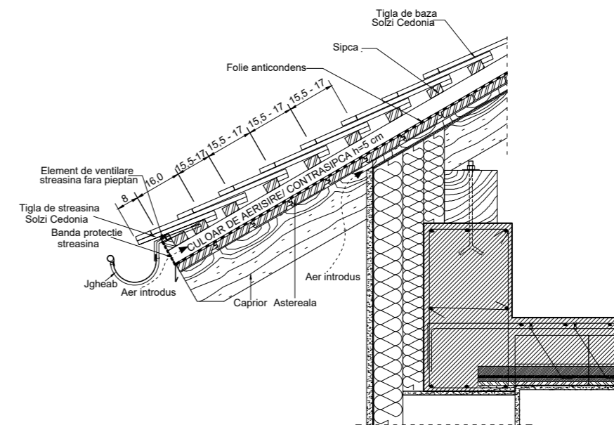
DETALIU STREAȘINĂ
