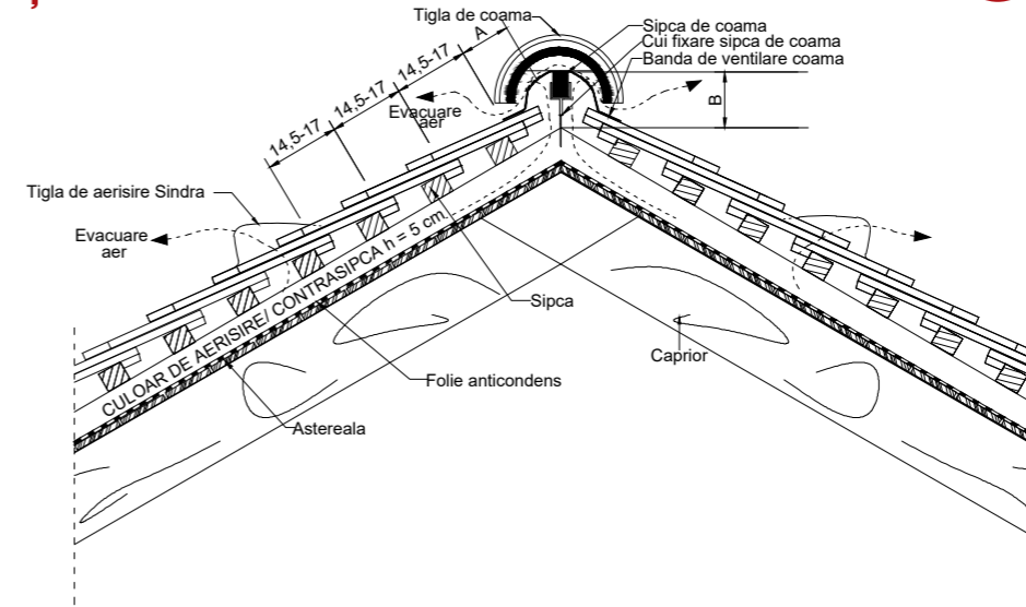
DETALIU COAMĂ
