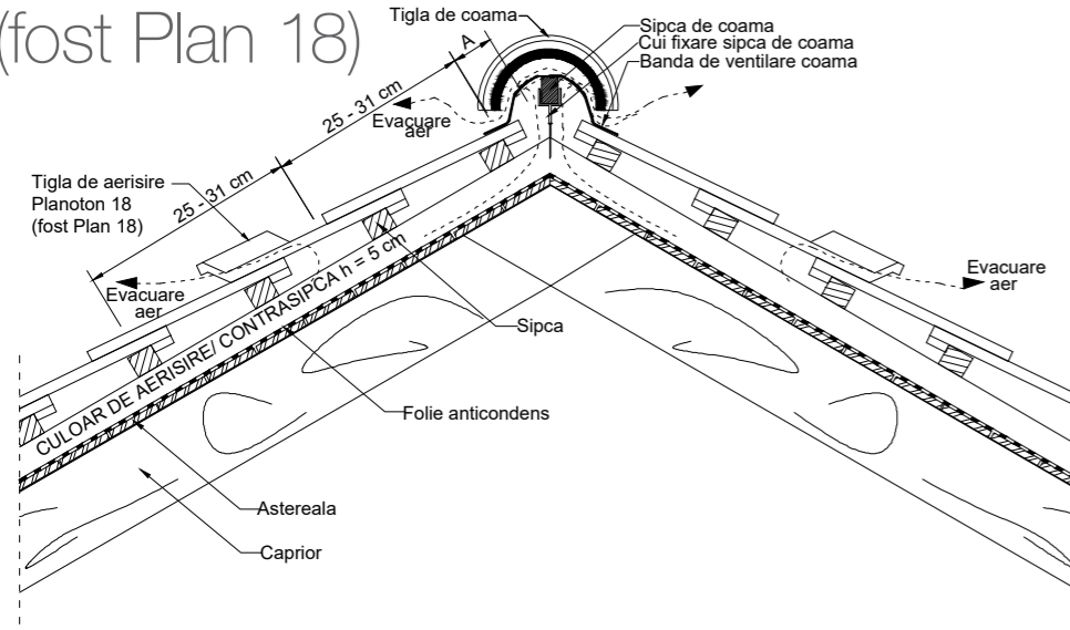
DETALIU COAMĂ
