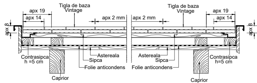
DETALIU ÎNCHIDERE MARGINE STÂNGA / DREAPTA
