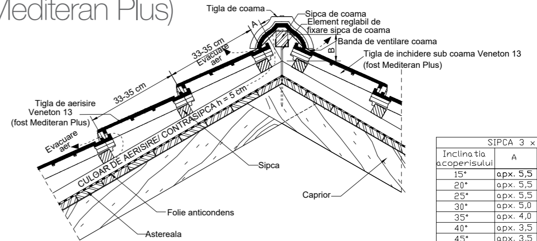
DETALIU COAMĂ
