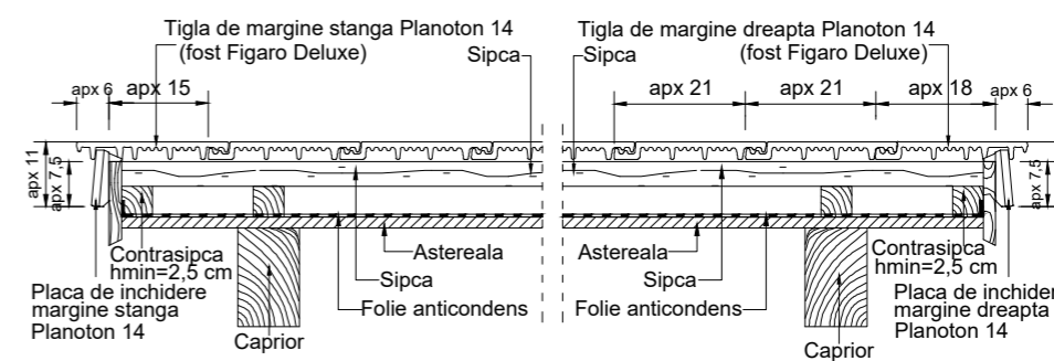
DETALIU ÎNCHIDERE MARGINE STÂNGA / DREAPTA
