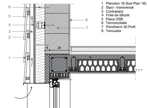
Detaliu 2
