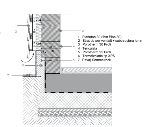
Detaliu 3
