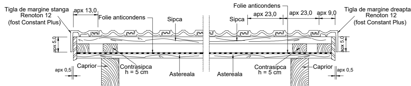
DETALIU ÎNCHIDERE MARGINE STÂNGA / DREAPTA
