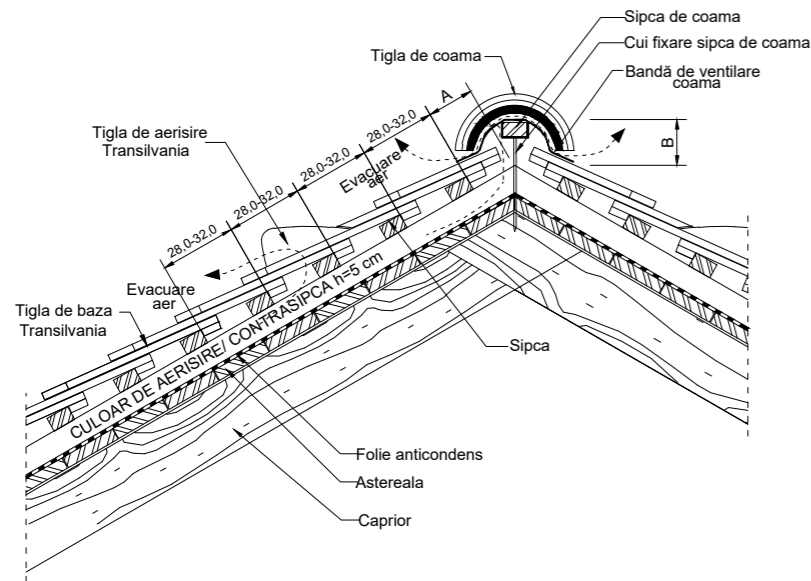
DETALIU COAMĂ
