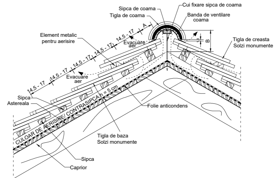
DETALIU COAMĂ
