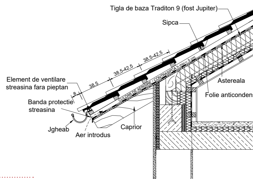
DETALIU STREAȘINĂ
