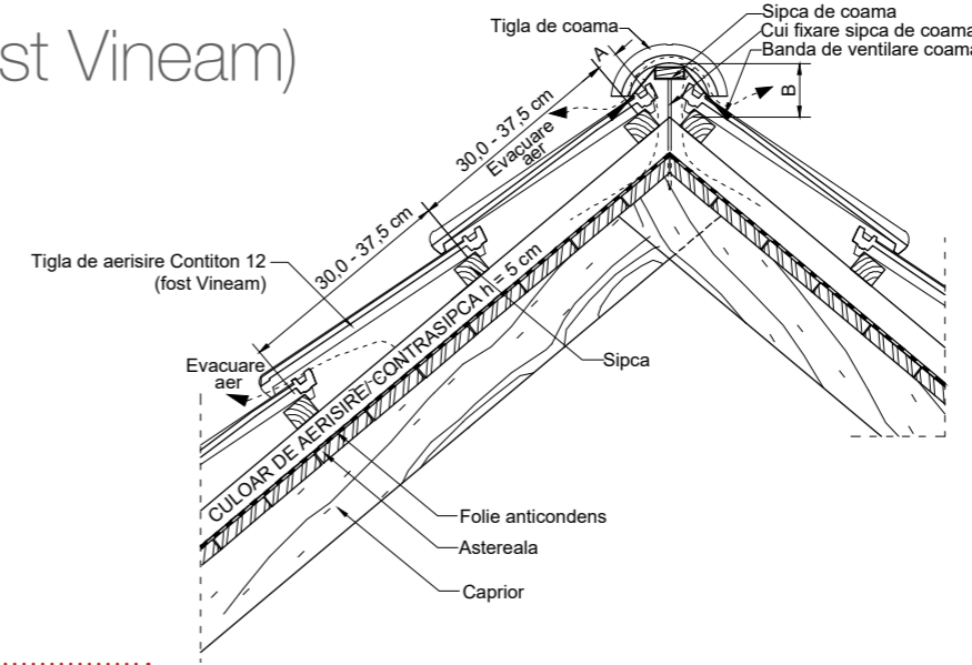
DETALIU COAMĂ
