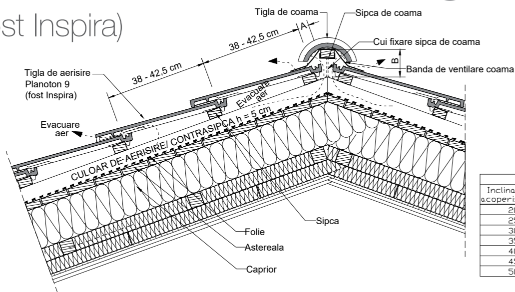
DETALIU COAMĂ
