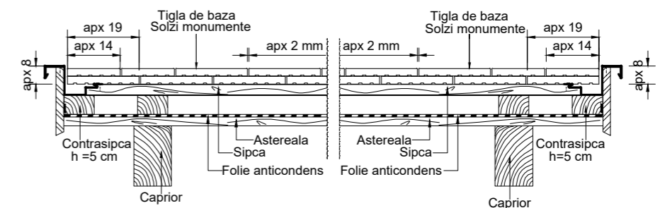
DETALIU ÎNCHIDERE MARGINE STÂNGA / DREAPTA
