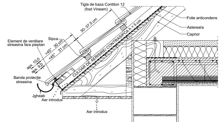
DETALIU STREAȘINĂ
