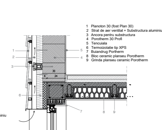
Detaliu 2
