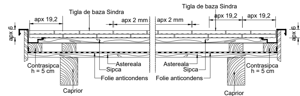
DETALIU ÎNCHIDERE MARGINE STÂNGA / DREAPTA
