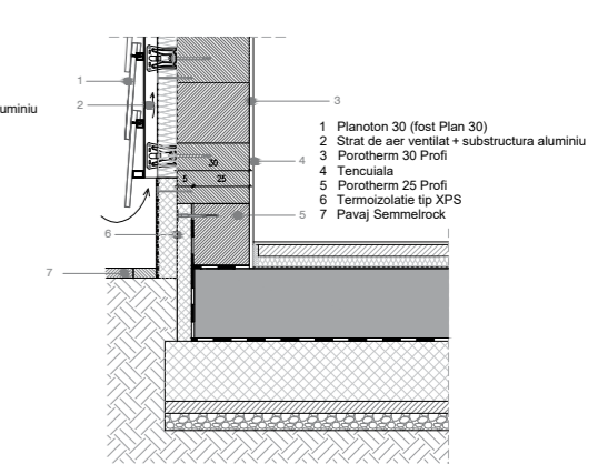
Detaliu 3
