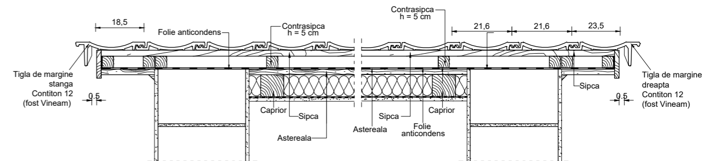
DETALIU ÎNCHIDERE MARGINE STÂNGA / DREAPTA
