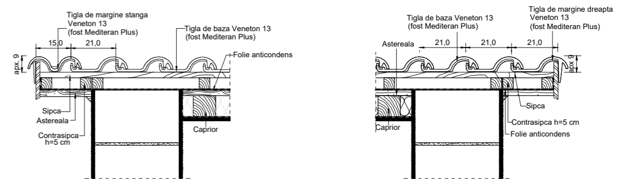
DETALIU ÎNCHIDERE MARGINE STÂNGA / DREAPTA
