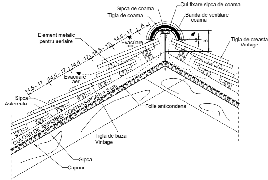
DETALIU COAMĂ
