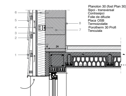
Detaliu 2
