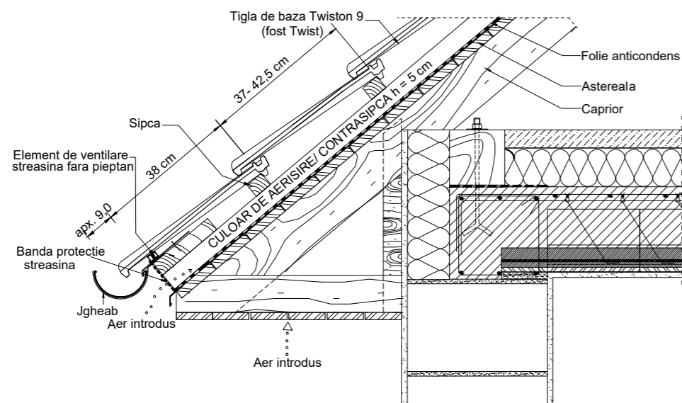
DETALIU STREAȘINĂ
