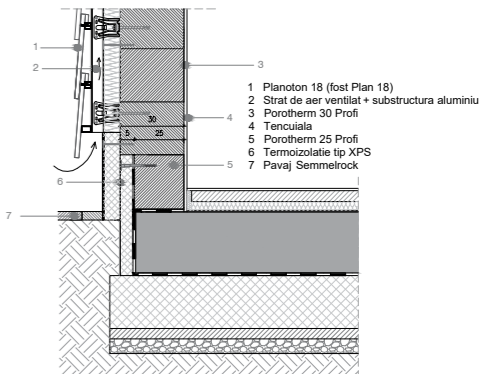
Detaliu 3
