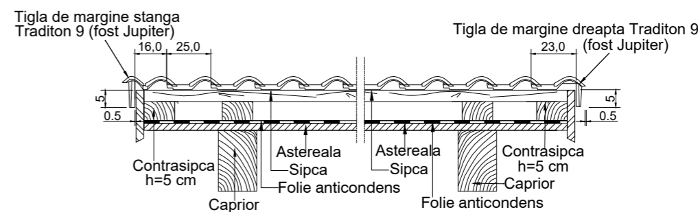
DETALIU ÎNCHIDERE MARGINE STÂNGA / DREAPTA
