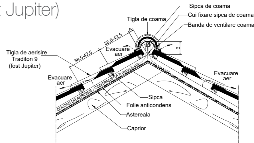
DETALIU COAMĂ
