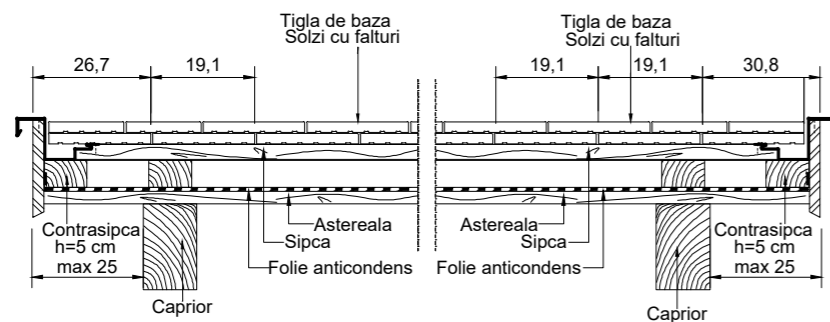
DETALIU ÎNCHIDERE MARGINE STÂNGA / DREAPTA
