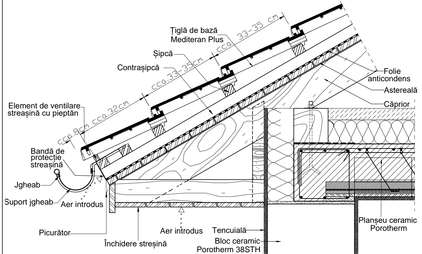
Țiglă ceramică Tondach - Detalii tehnice
