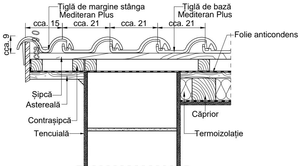
Detaliu de margine stânga
