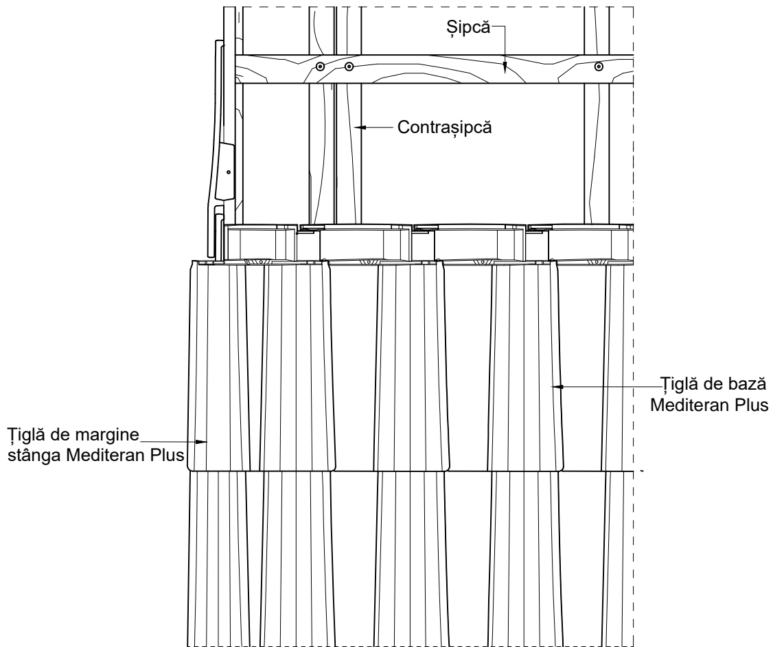
Detaliu de margine stânga
