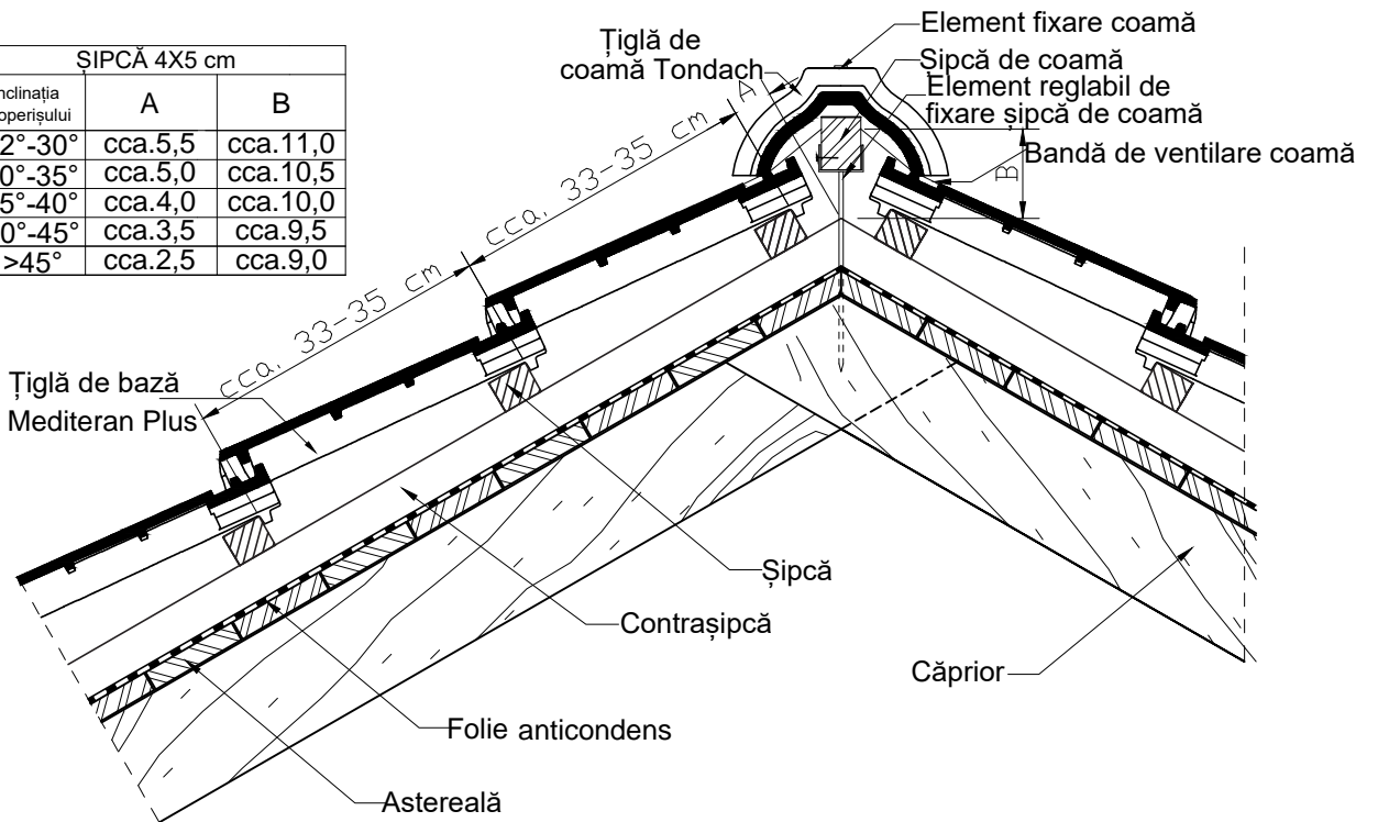
Țiglă ceramică Tondach - Detalii tehnice
