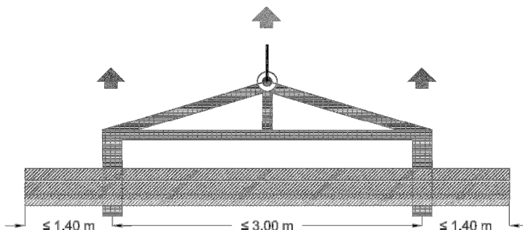
FIG.2 CONDIȚII GENERALE DE RIDICARE CU UTILAJ PREVĂZUT CU MACARA (grinzi de planșeu Porothersm și buiandrugi Porothersm)
