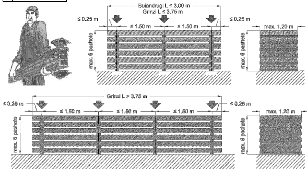
FIG.2 CONDIȚII GENERALE DE RIDICARE CU UTILAJ PREVĂZUT CU MACARA (grinzi de planșeu Porothersm și buiandrugi Porothersm)
