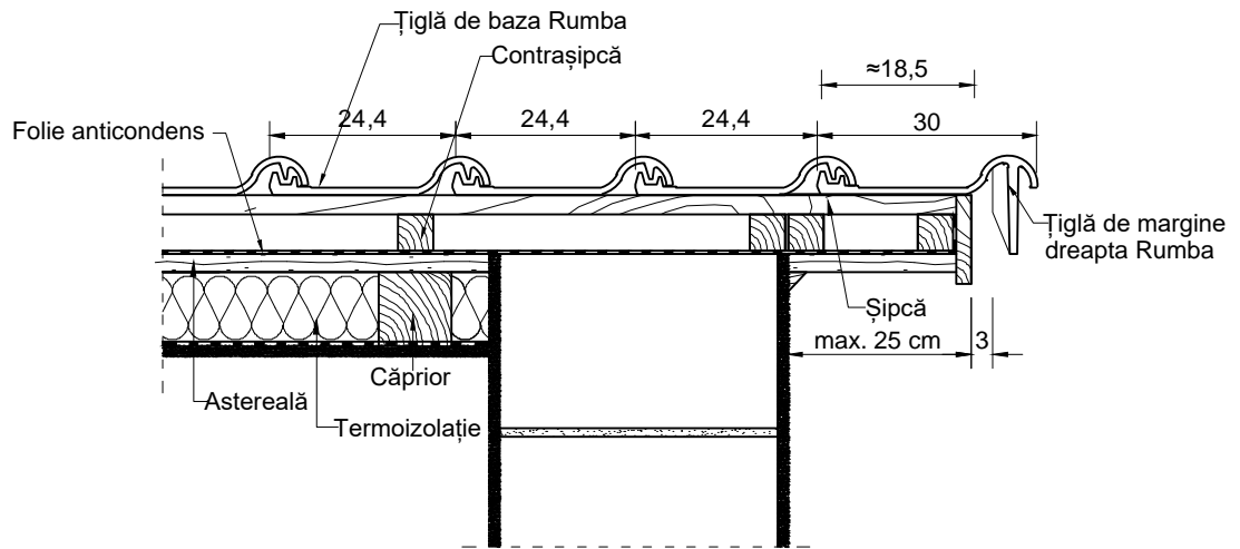
Detaliu de margine dreapta
