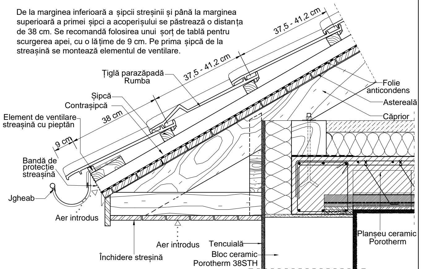
Țiglă ceramică Tondach - Detalii tehnice
