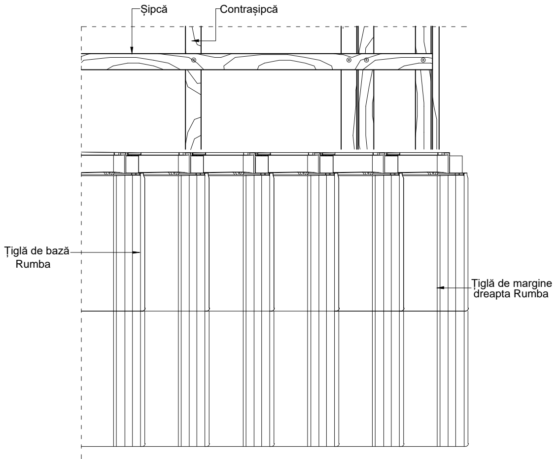
Detaliu de margine dreapta
