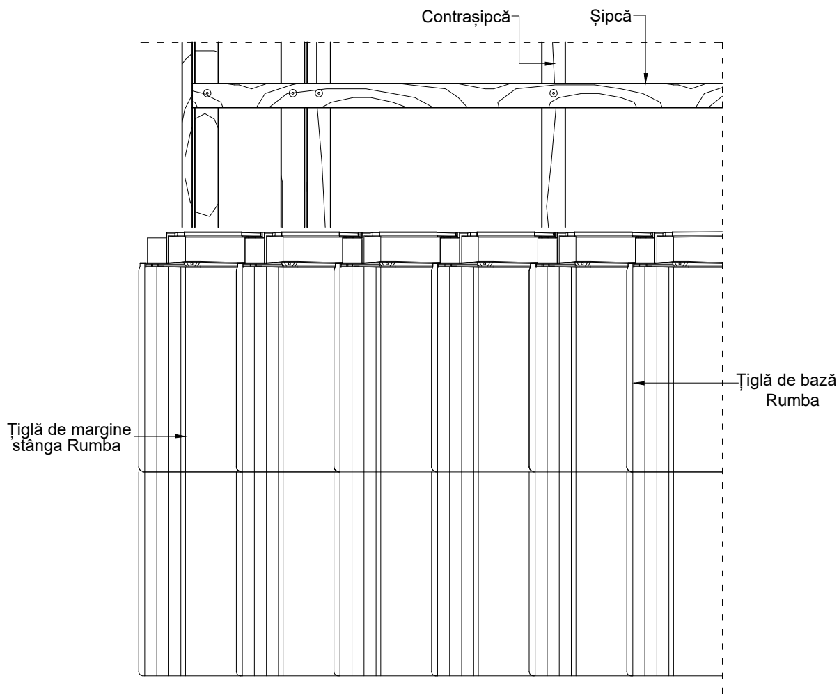
Detaliu de margine stânga
