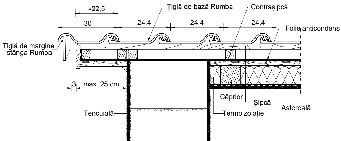
Țiglă ceramică Tondach - Detalii tehnice
