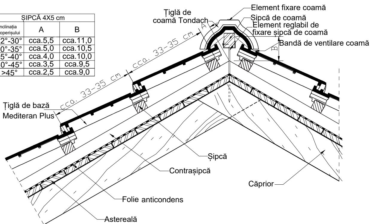
Țiglă ceramică Tondach - Detalii tehnice
