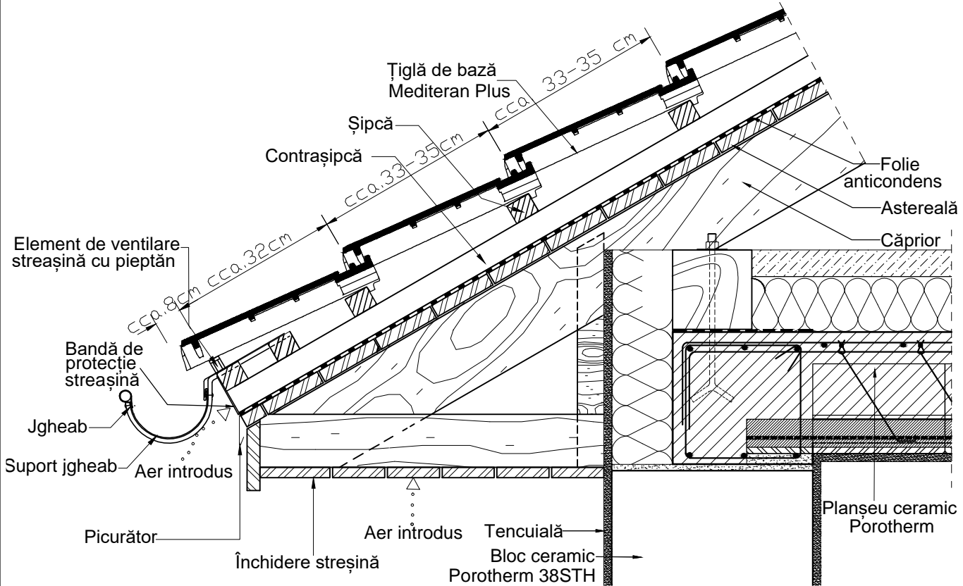
Țiglă ceramică Tondach - Detalii tehnice
